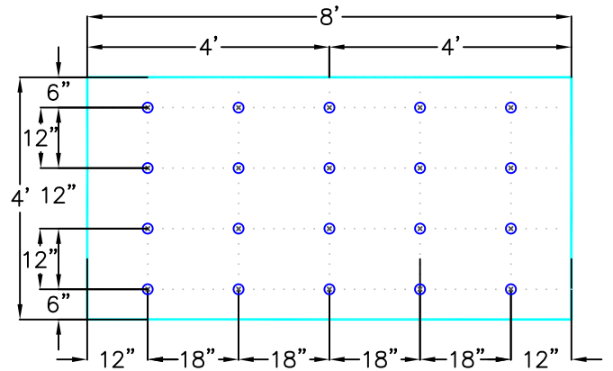
20 FASTENERS PER 4'x8' BOARD
