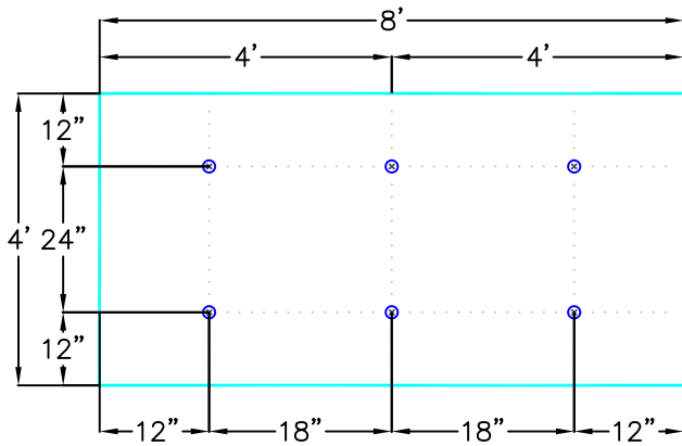
6 FASTENERS PER 4'x8' BOARD
