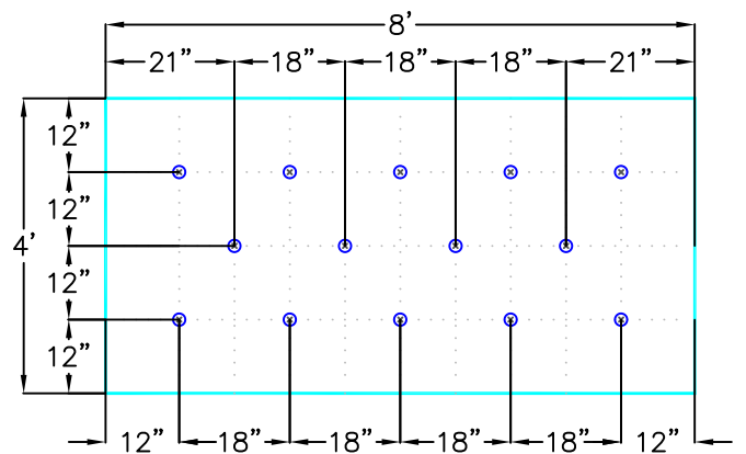
14 FASTENERS PER 4'x8' BOARD
